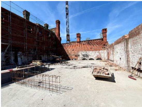
1. Obergeschoss - die Dachstuhlträger wurden bereits entfernt
