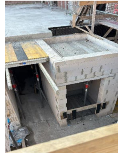
Aufzug mit Anbindung Boden im Erdgeschoss
